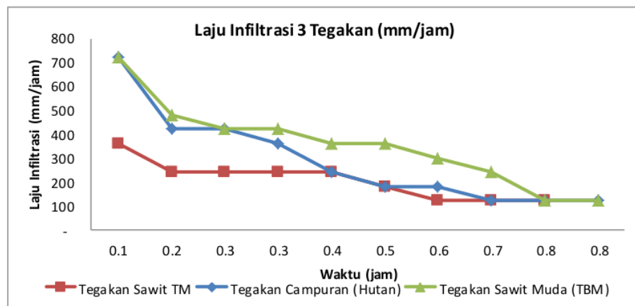
Gambar 1. Grafik Laju Infiltrasi Tiga Tegakan
