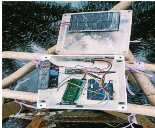
Gambar 1.2 Alat ukur tinggi muka air otomatis (AWLR).
