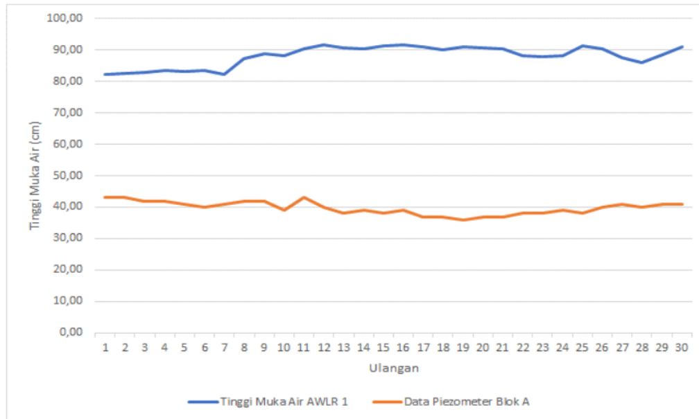
Gambar 4.15 Grafik Fluktuasi Data AWLR 1 dan Piezometer Blok A
