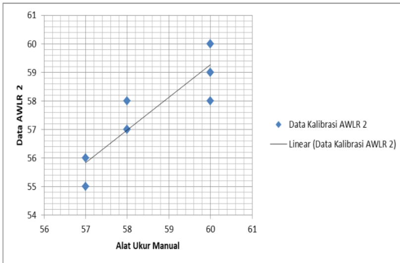
Gambar 1.12 Grafik Scatter Kalibrasi AWLR 2 Blok B
