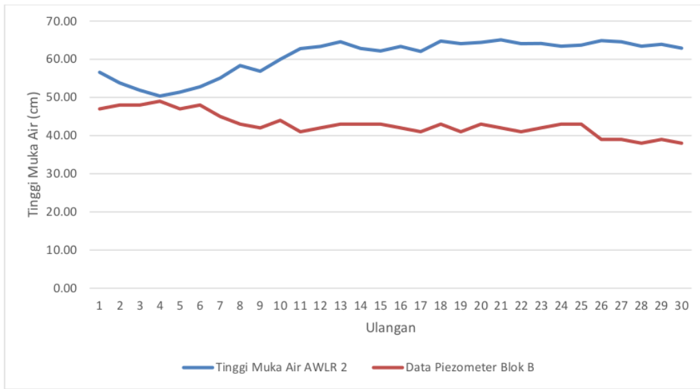
Gambar 1.16 Grafik Fluktuasi Data AWLR 2 dan Piezometer Blok B
