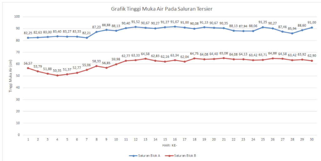
Gambar 1.12 Grafik Fluktuasi Harian AWLR 1 Blok A dan AWLR 2 Blok B
