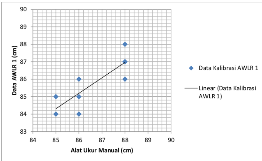
Gambar 1.11 Grafik Scatter Kalibrasi AWLR 1 Blok A
