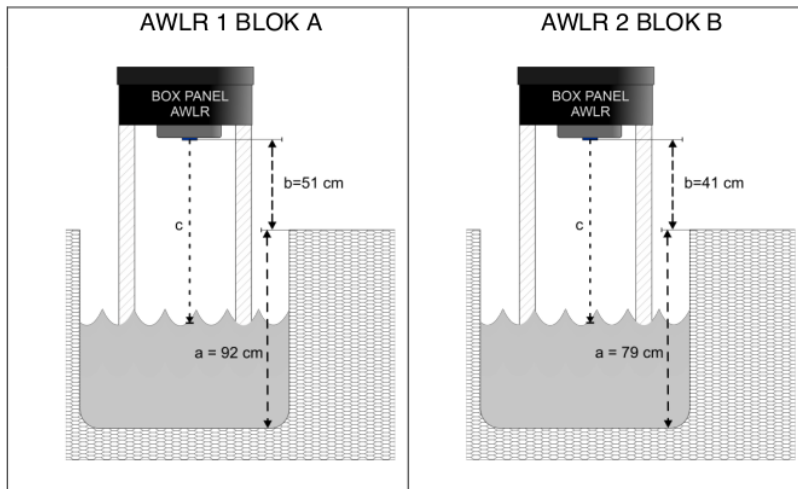
Gambar 1.10 pengukuran kedalaman saluran dan tinggi AWLR.
