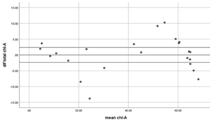
Gambar 4.2 Rentang kesesuaian antara total klorofil laboratorium dengan fitur warna A ( mean chl-A : nilai tengah antara total klorofil dengan fitur warna A, diff total chl-A : rentang perbedaan dari pengukuran antara total total klorofil dengan fitur warna A)
