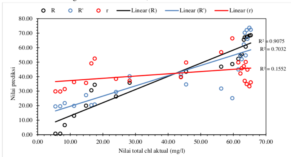
Grafik 4.6 Nilai prediksi total chl dengan fitur R , R' dan r
