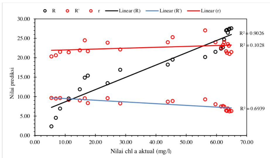
Grafik 4.2 Nilai prediksi chl a dengan fitur R , R' dan r
