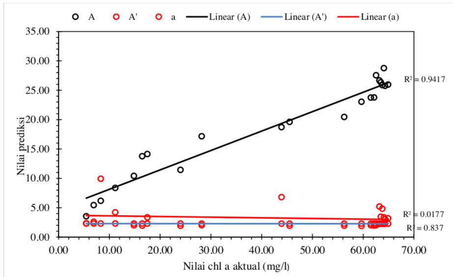
Grafik 4.1 Nilai prediksi chl a dengan fitur A , A' dan a
