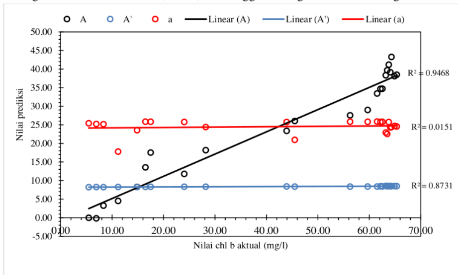
Grafik 4.4 Nilai prediksi chl b dengan fitur A , A' dan a
