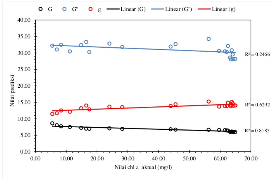
Grafik 4.3 Nilai prediksi chl a dengan fitur G , G' , dan g
