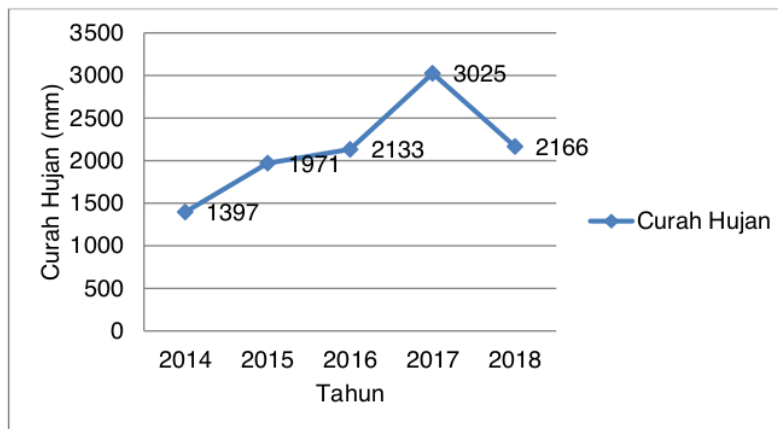
Gambar 1. Grafik curah hujan tahun 2014 – 2018
