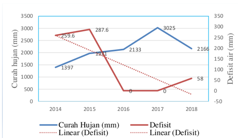
Gambar 2. Grafik curah hujan dan defisit air 2014 - 2018
