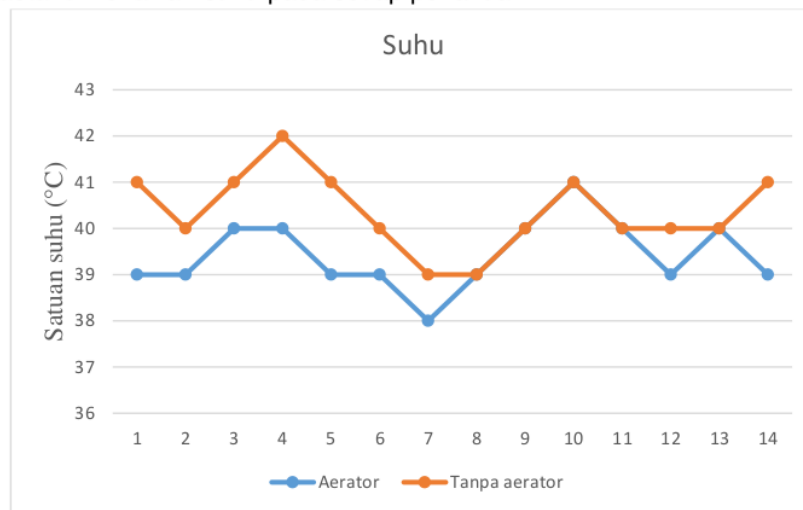
Gambar 6. analisa Grafik Suhu Menggunakan dan Tanpa Aerator
