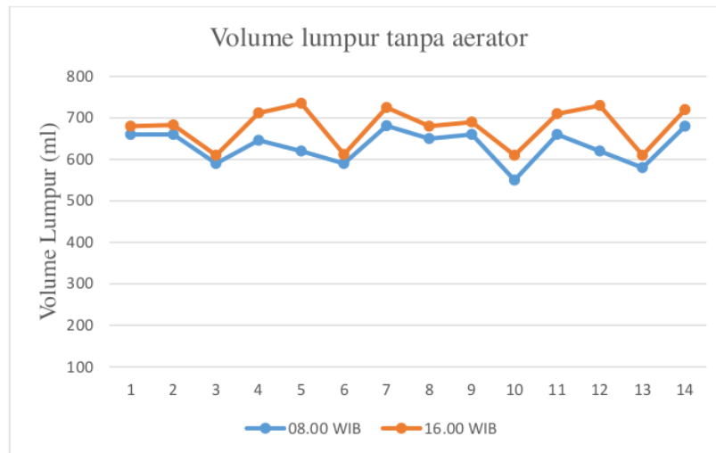
Gambar 8. Volume lumpur kolam tanpa aerator
