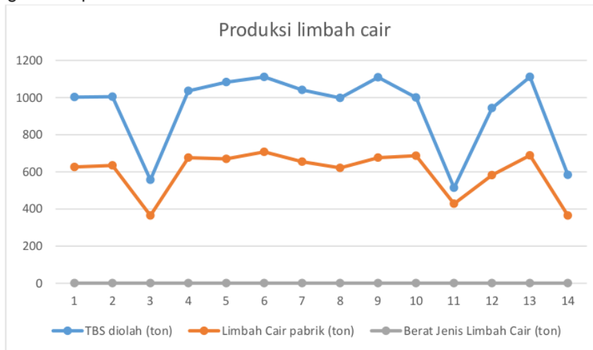
Gambar 4. Produksi limbah cair di bulan Agustus
