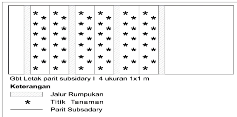
Gambar 4.2. Dena lokasi saluran tersier dengan pola 4:1
