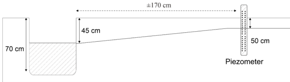
Gambar 4.12. Posisi piezometer dari saluran tersier
