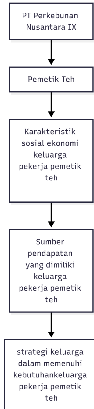
Gambar 2.1 kerangka pemikiran
